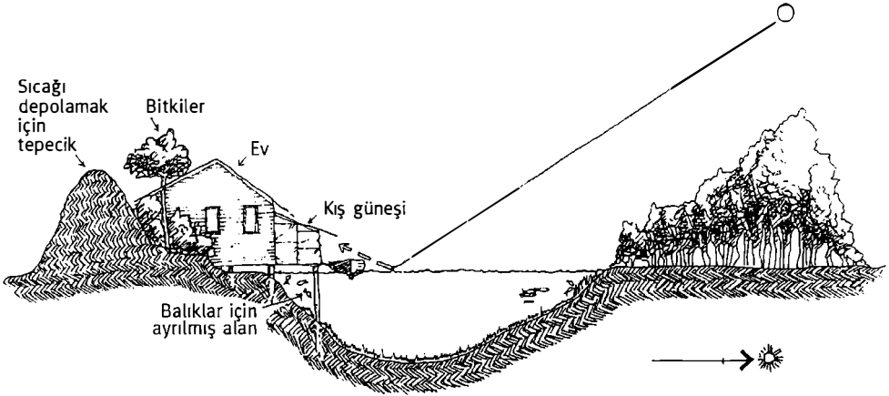
ŞEKİL 2.8 Kış güneşini yansıtan kütleler olarak göletler veya su bentleri, sabah, öğlen veya kış ısını artırarak seralar ve ekili alanlar için faydalı olur (güneş gören tepecikler özel olgunlaştırma alanlarıdır).
